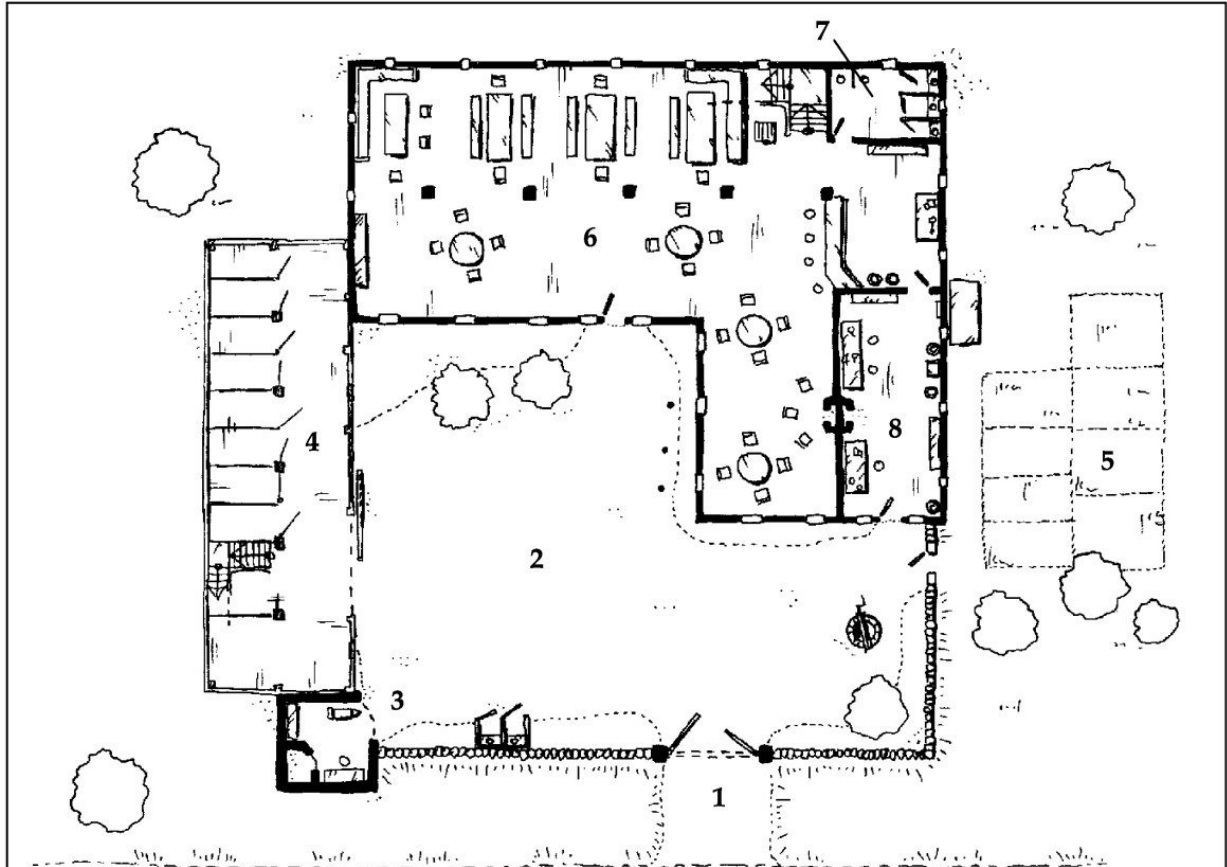
Erdgeschoß
